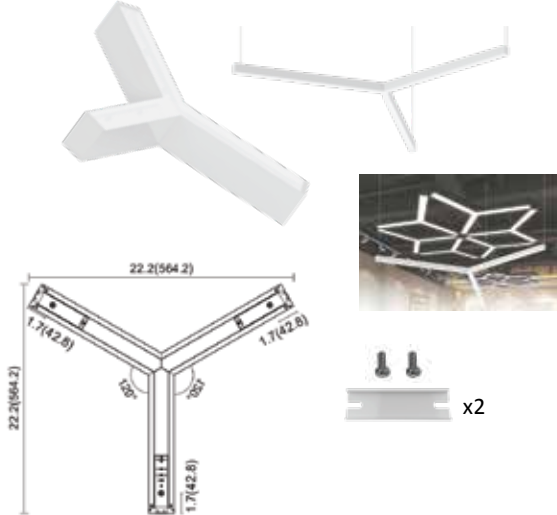
Y Connector
